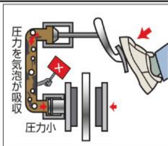
<ベーパーロックによるブレーキ性能低下>
